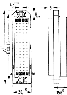
Federleiste 72polig
