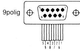
Buchsenleisten
