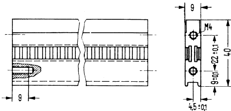
Tragschiene, hinten innen
