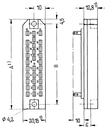
Federleiste 30polig
