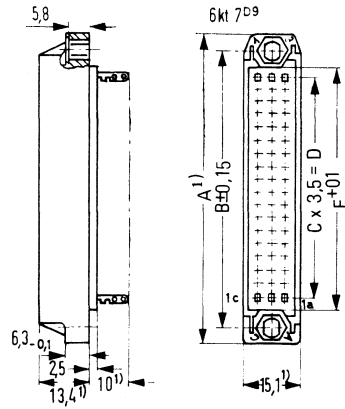
Messerleiste 72polig
