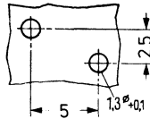
Montagelochung (Bauteilseite)
