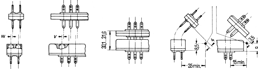
Zulässige Mittenabweichungen in mm
