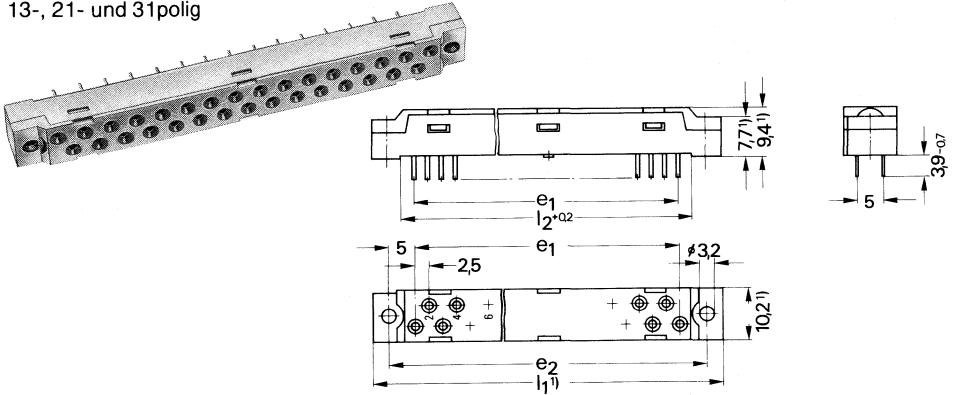
Montagelochung (Bauteileseite)
