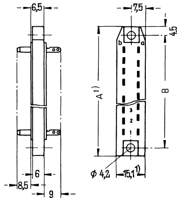
Messerleiste 30polig
