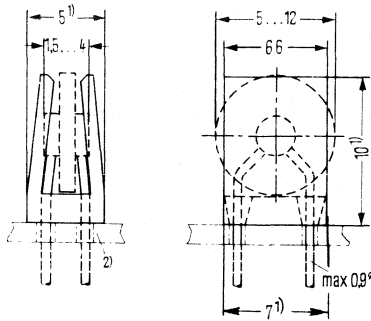
Montagelochung (Bauteilseite)
