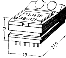
Form rechteckig mit 2 Leuchtdioden
