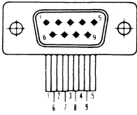
Stiftleisten
