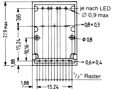
Form rechteckig mit 2 Leuchtdioden
