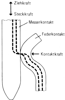
Bild. Durch Einschnüren der Stromfäden im Kontaktbereich wird der Engewiderstand R_E verursacht.
