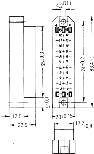
Federleiste 39polig
