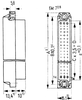
Messerleisten 21- bis 54polig
