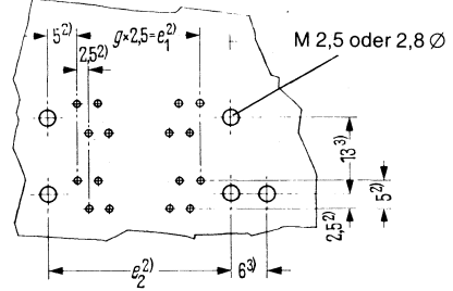
Montagelochung (Bauteileseite)
