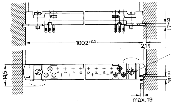
Leiste teilbestückt
