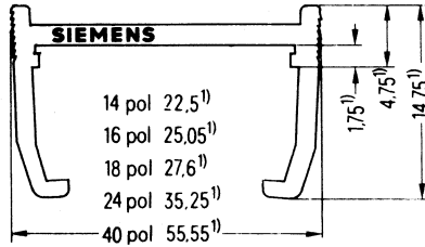
Verriegelungsbügel
