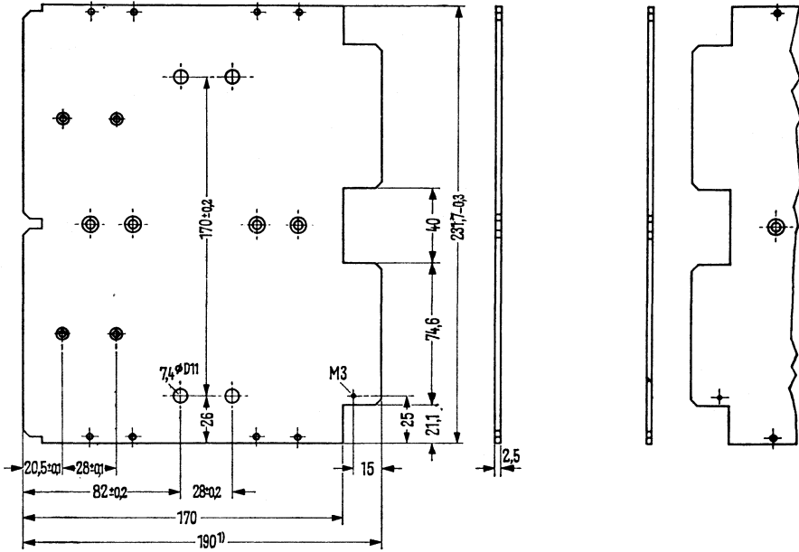
Seitenteil rechts
