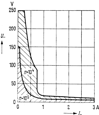
Kontakteile versilbert
