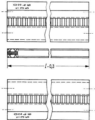
Tragschiene, vorne innen
