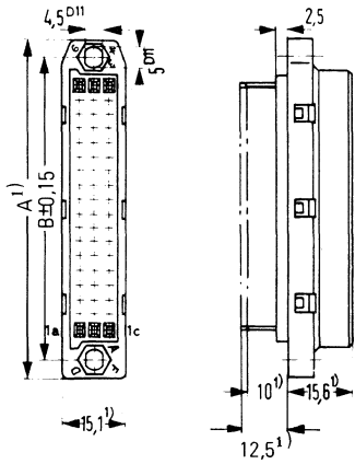
Federleiste 72polig
