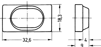
Kappe 1 3/4 fach
