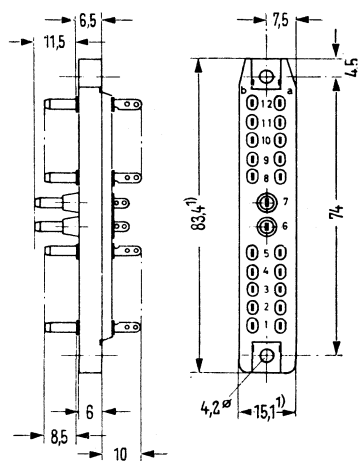
Messerleiste
