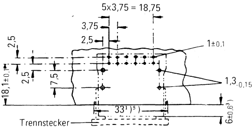
Montagelochung (Bauteileseite)
