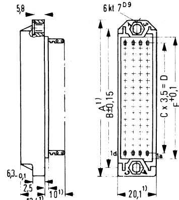
Messerleiste 72polig
