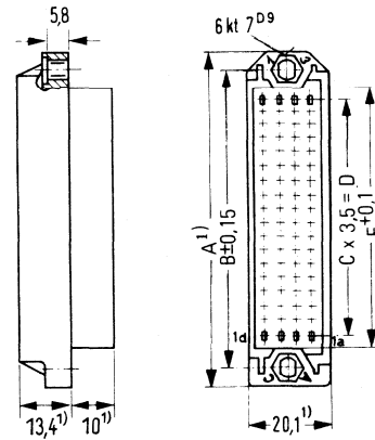
Messerleiste 72polig
