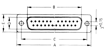
Buchsenleiste 9- bis 37polig
