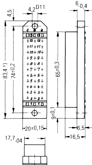
Messerleiste 39polig
