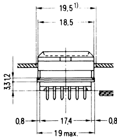
Form quadratisch ohne Leuchtdiode
