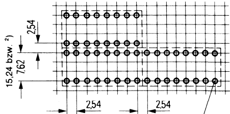
Rasterlochung (Bauteilseite)
