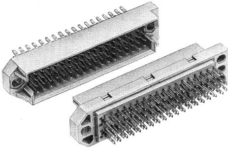
mit Lötösen
