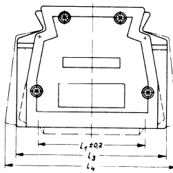
Gehäuse mit eingesetzten Rastbügeln
