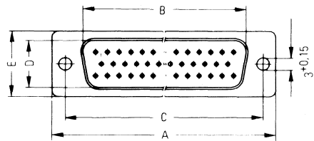
Buchsenleiste 50polig
