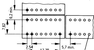
Rasterlochung (Bauteileseite)
