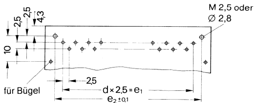
Montagelochung (Bauteilseite)
