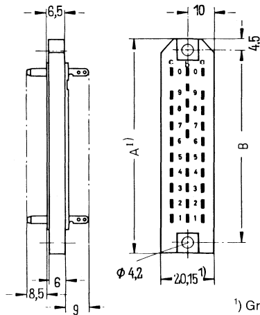
Messerleiste 30polig
