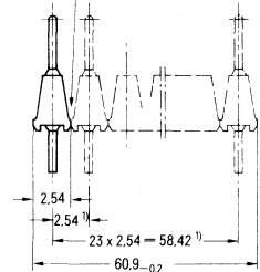
Verbindungen abtrennbar
