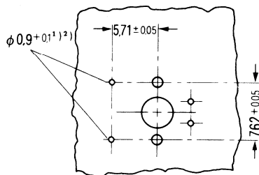
Zusatzlochung für Schaltdiode BAW 75, falls eingebaut (nur für Varianten »Schließer tastend« möglich)
