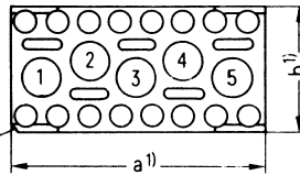
Identifikations- facette für Kontakt 1
