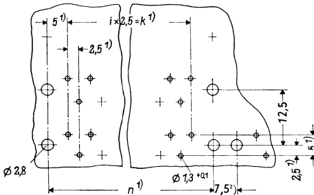
Montagelochung (Bauteileseite)
