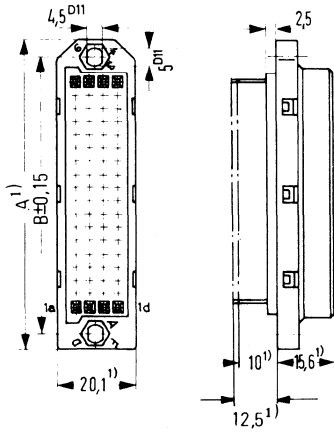
Federleiste 72polig
