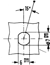
Montagelochung
