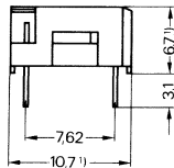
Unterteil
