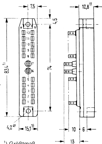
Federleiste
