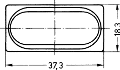
Kappe 2fach
