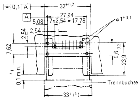
Montagelochung (Bauteileseite)
