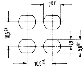
Montagelochung (Beispiel für 4 Drucktasten)
