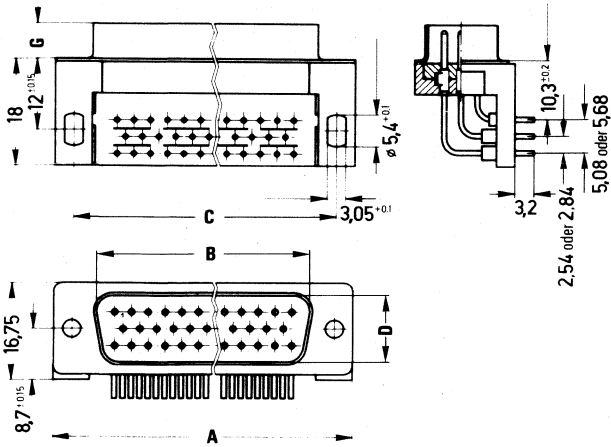
Winkelstecker Buchsenleiste 50polig
