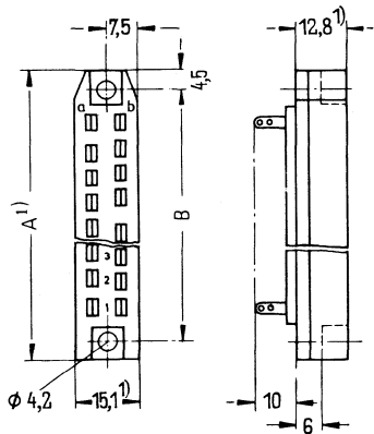
Federleiste 30polig
